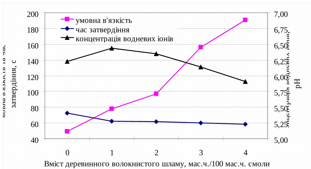
Рис. 1. Вплив вмісту волокнистого шламу на умовну в'язкість, час затвердіння та концентрацію водневих іонів (рН) клею
