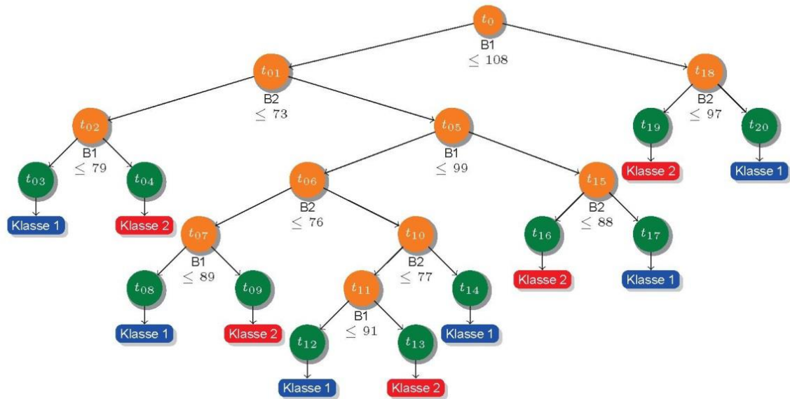
Рис. 3. Приклад дерева рішень для набору даних з двома змінними, що поділяють на два класи
