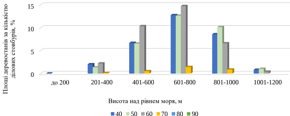
Рис. 5. Структура модальних букових деревостанів за кількістю ділових стовбурів і висотою над рівнем моря в межах Вулканічних Українських Карпат (a) і південного мегасхилу Полонинського хребта (b) Fig. 5. Structure of modal beech stands by the number of merchantable trunks and altitude above sea level within the Volcanic Ukrainian Carpathians (a) and the southern megaslope of the Polonynian Ridge (b)
